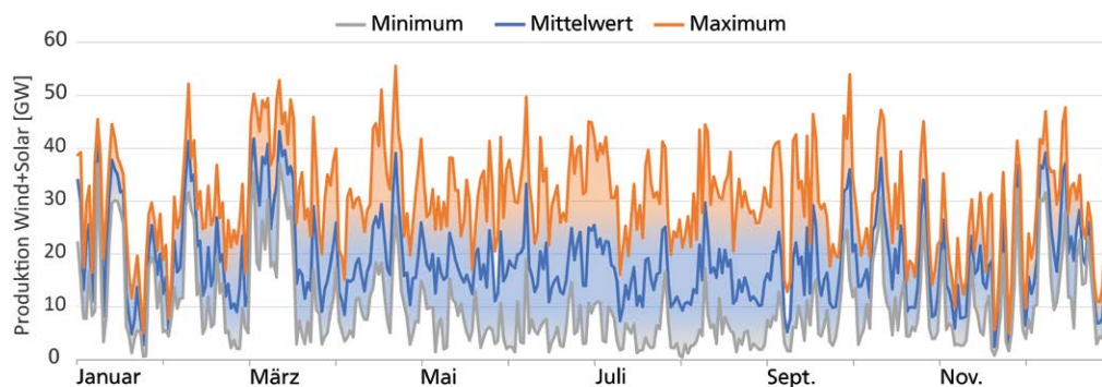
Abb. 2: Stundengemittelte Stromerzeugung aus Windkraft und Photovoltaik in Deutschland im Jahr 2019. Daten aus [En]. Die Frequenz der Schwankungen ist in den Wintermonaten besonders ausgeprägt.
