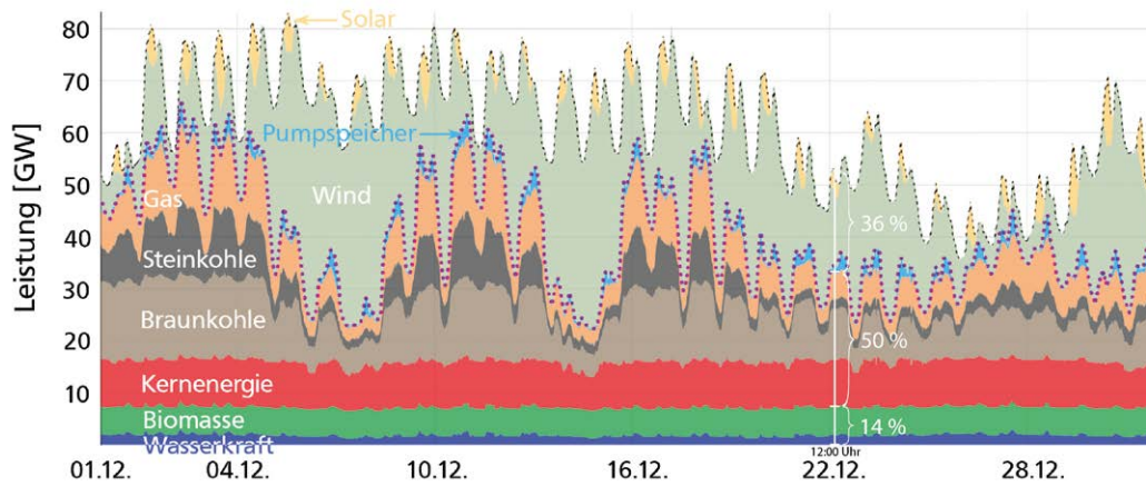
Abb. 3: Stromerzeugung aus unterschiedlichen Quellen und zeitlich fluktuierender maximaler Leistungsbedarf (obere, graue Punktlinie) im Dezember 2019 in Deutschland; reproduziert nach [Ent]. Der Öl-Anteil ist wegen seiner Geringfügigkeit nicht dargestellt. Die untere gepunktete Linie (magenta) markiert den Leistungsbeitrag von Wasserkraft, Biomasse, Kernenergie, Stein- und Braunkohle, Gas sowie Pumpspeicher. Die Differenz zur zeitlich fluktuierenden Gesamtleistung ergibt den Anteil von Wind- und Sonnenenergie. Das Beispiel für den 22. Dezember 2019 zur Mittagszeit weist einen Anteil von Wind- und Solarenergie von circa 36 Prozent aus.
