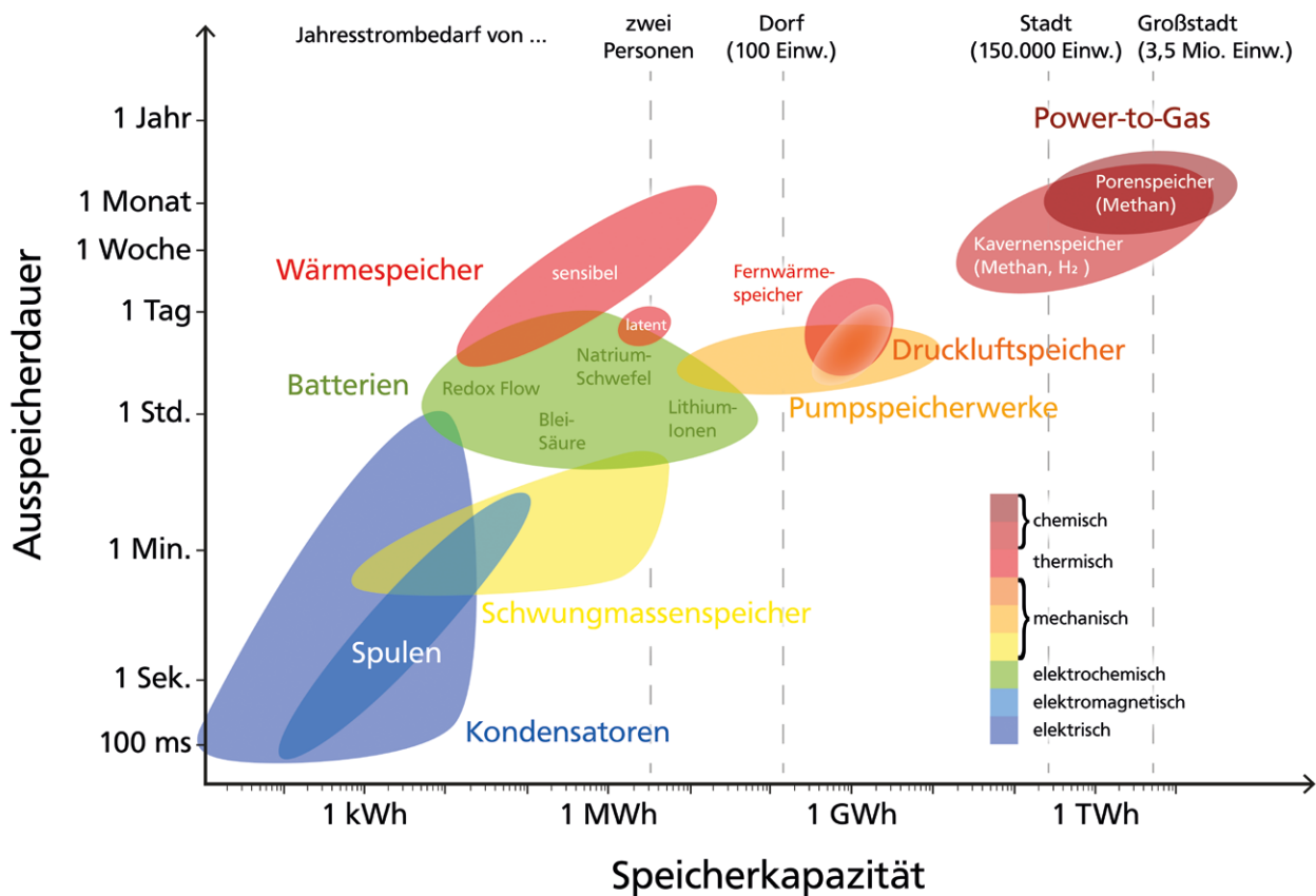
Abb. 1: Speicherkapazität und Ausspeicherdauer verschiedener Speichertechnologien im Überblick. Reproduziert nach [St14].
