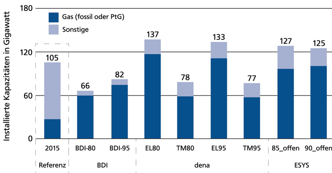
Abb. 4: Szenarien für den Bedarf an regelbaren Kraftwerkskapazitäten in Deutschland im Jahr 2050, reproduziert nach [De19]. Dort werden die Szenarien auch detailliert erläutert.
